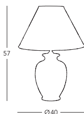
■ 0014.74.3 Tischleuchte / table lamp ☑ 1 lp., E27, 100W / LED E27 Lampenschirm / lampshade 0014.S02 ☑ 40 cm, ☐ 25 cm
